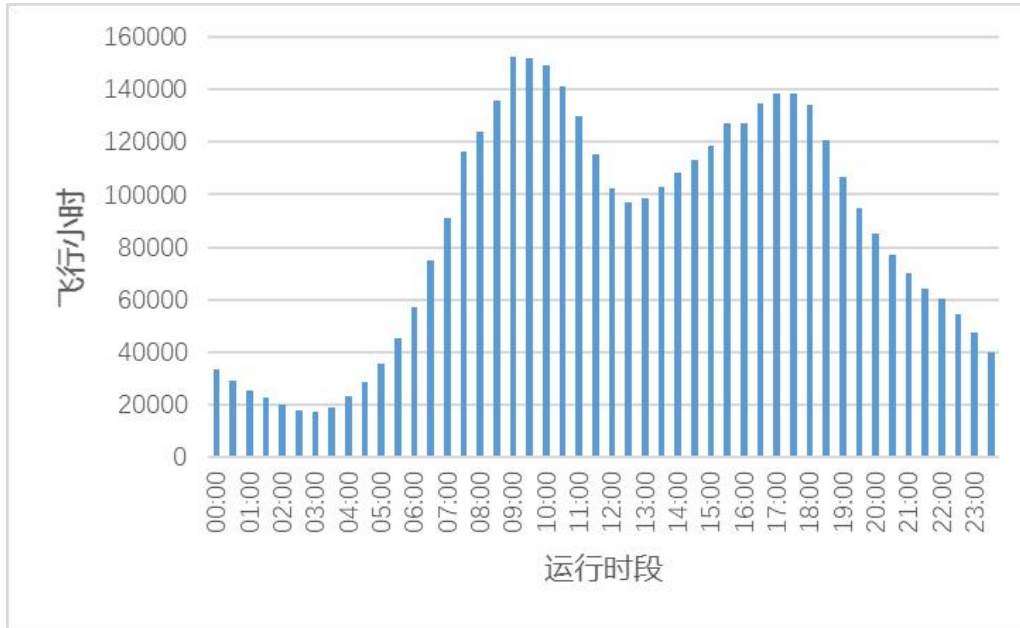
图 4-4 2023 年无人机运行时段分布
